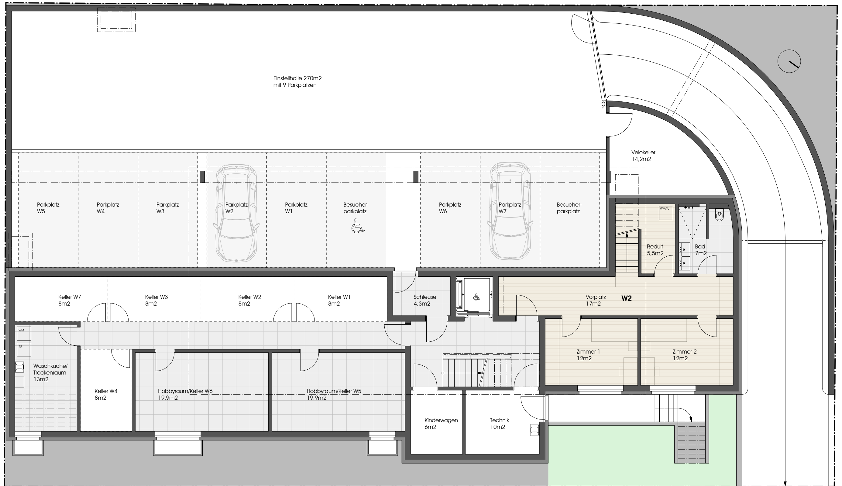
Grundriss Untergeschoss
